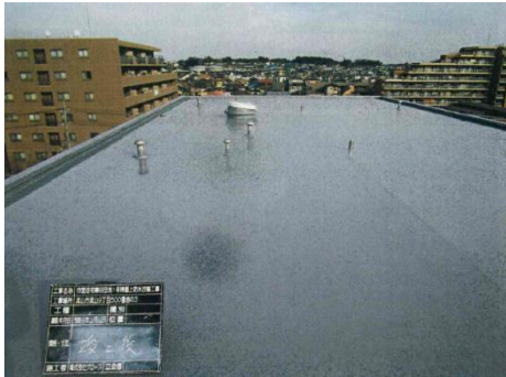
屋上防水工事を実施した柳田団地1号棟
